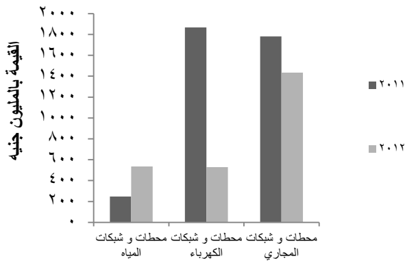
ما تم تنفيذه من محطات وشبكات بواسطة شركات القطاع الخاص
