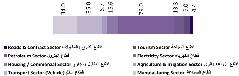
نسبة الإنبعاآت من ثاني اكسيد الكربون 2013/12 Percentage of Emissions of Co2 12/2013
